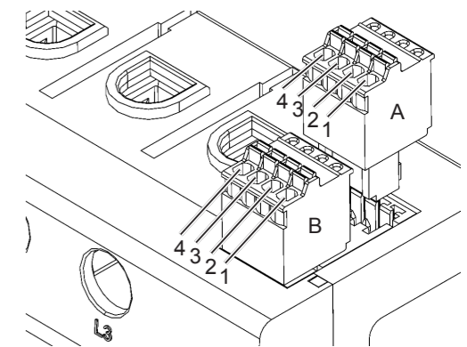
Anschlussplan für RS485-Stecker:
